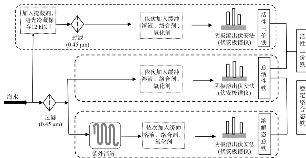
图4 海水中不同形态铁的检测流程
